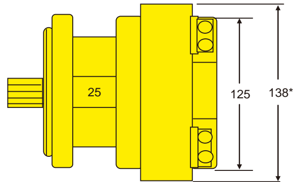
俯视图
