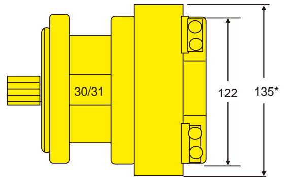
俯视图
