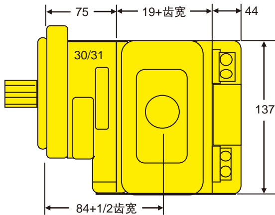
主视图
