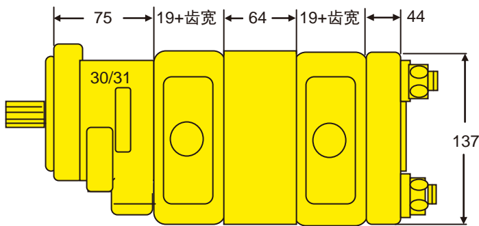
主视图
