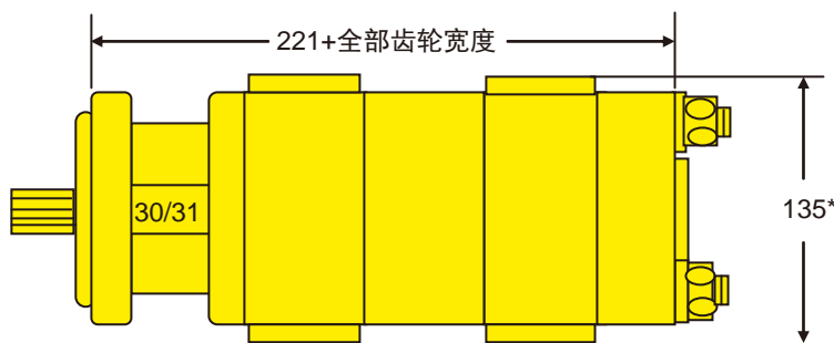
俯视图
