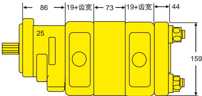
主视图
